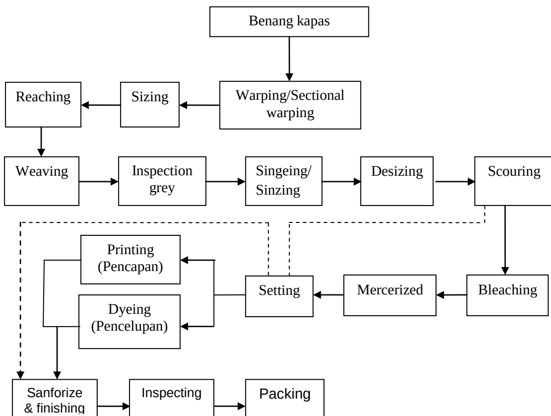
Gambar 2. Flow-Chart Proses Produksi Kain tenunan dari kapas
