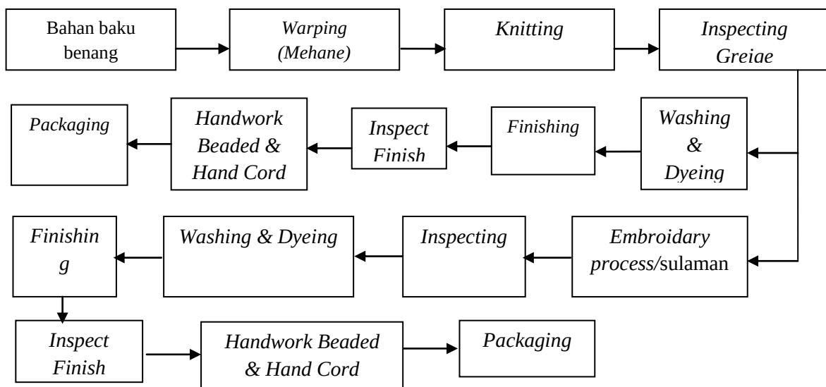
Gambar 8. Flow-Chart Proses Produksi Kain Tenunan Khusus dan Sulaman
