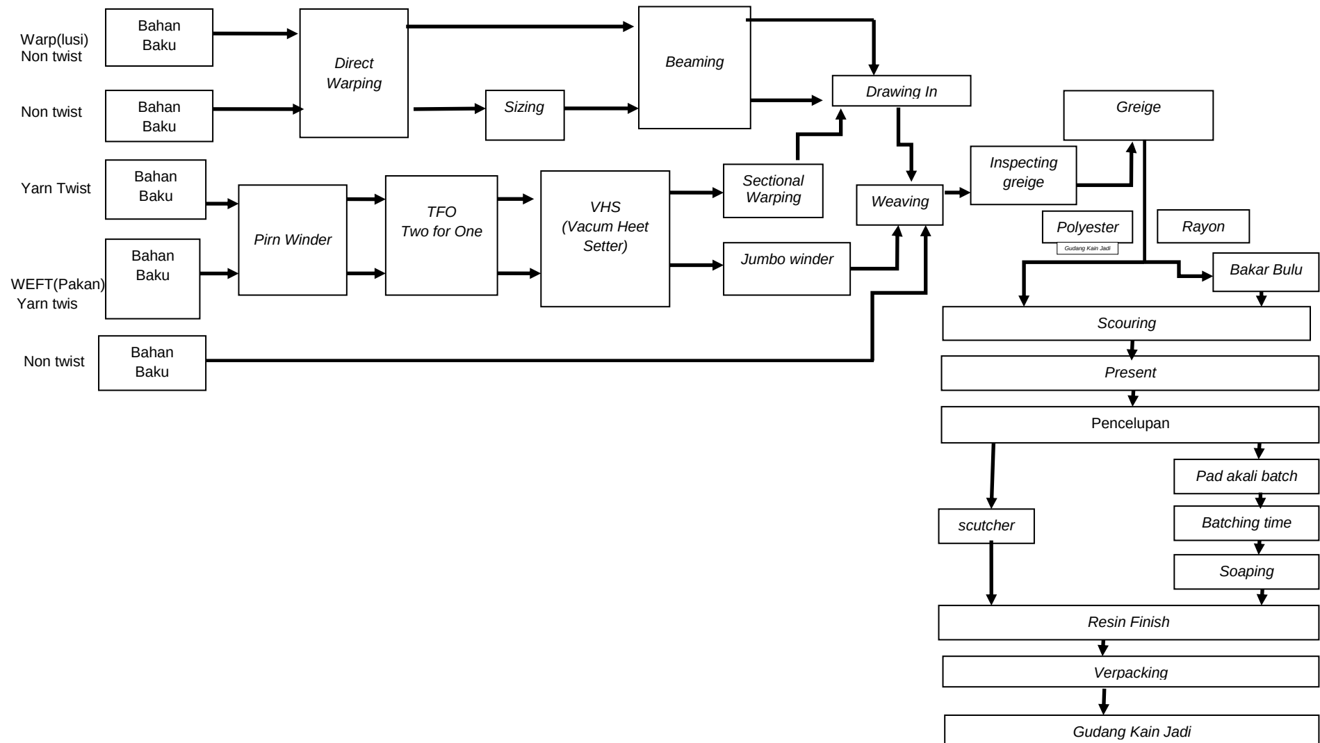
Gambar 6. Flow-Chart Proses Produksi Tenunan Dari Benang Filamen Sintetik Dan Artifisial, Pemohon
